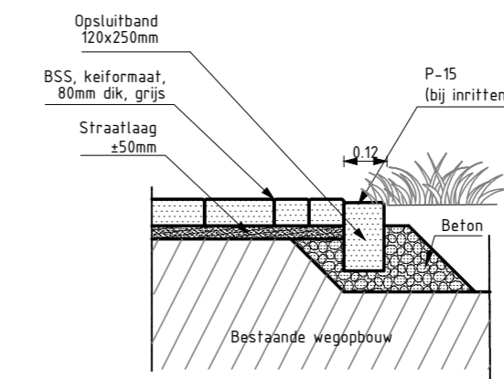
OPSLUITBAND LANGS RIJBAAN
