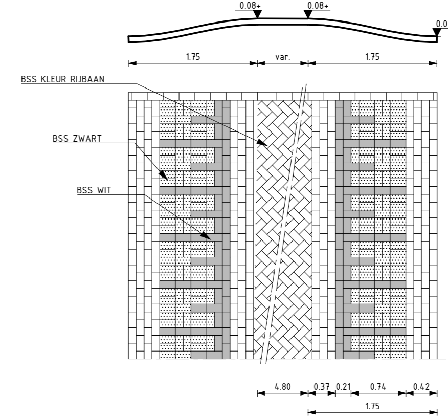
DREMPEL BIJ KOMGRENS 8cm 30KM/uur
