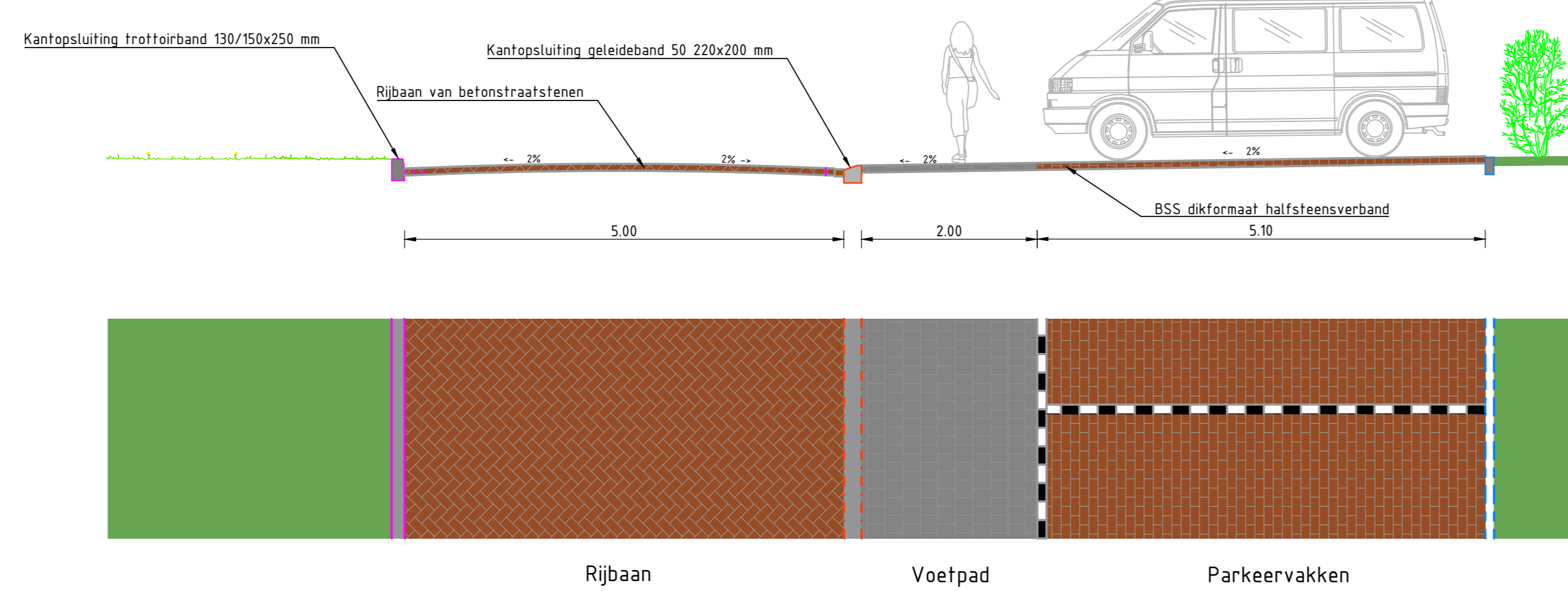
Doorsnede A-A met bovenaanzicht
