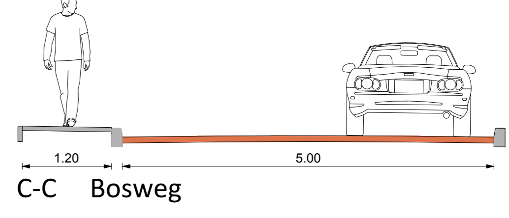
Dwarsprofielen Klarenbeek
